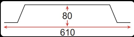
PVT1 L: 610mm W: 610mm
