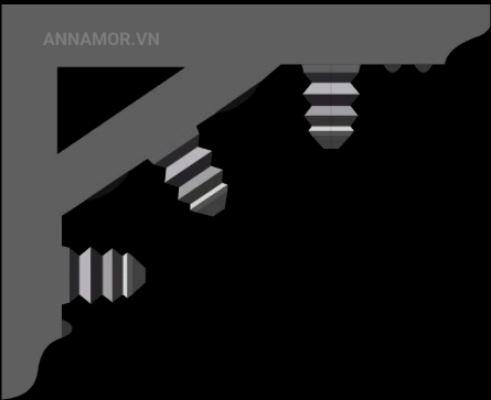
CGMB26A H: 250mm W: 350mm CGMB26B H: 300mm W: 400mm CGMB26C H: 350mm W: 450mm CGMB26D H: 400mm W: 500mm CGMB26E H: 500mm W: 600mm
