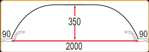
PVT15 D: 2000mm
